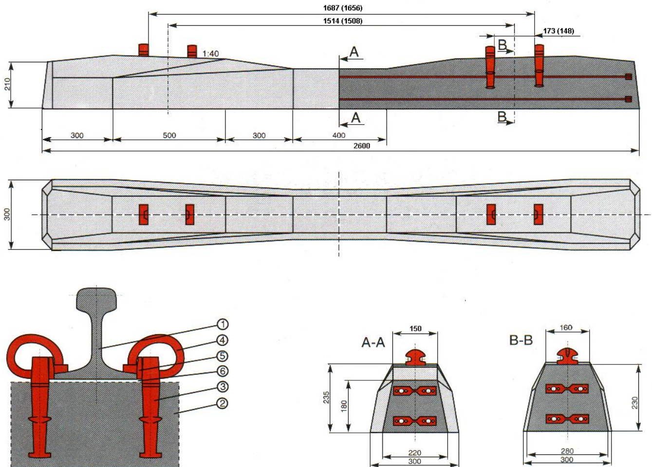
PRZYTWIERDZENIE SPRĘŻYSTE SB-3
