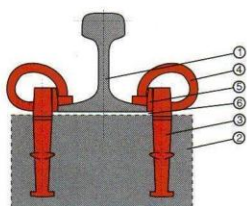
PRZYTWIERDZENIE SPRĘŻYSTE SB-3
