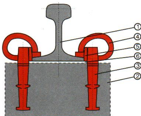
PRZYTWIERDZENIE SPRĘŻYSTE SB-3
